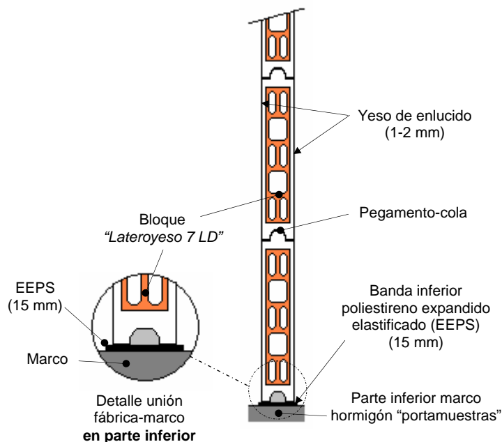
Figura 1: Esquema de muestra ensayada (B0812-46-M79)
